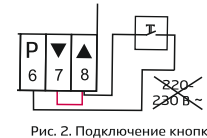
Рис. 2. Подключение кнопки
