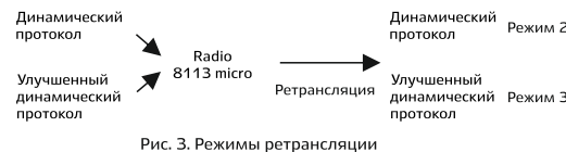
Рис. 3. Режимы ретрансляции
